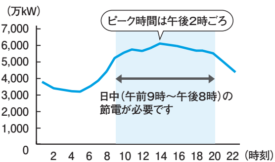
グラフ1 夏の1日の電力需要(最大電力需要発生日) 参考:資源エネルギー庁推計
