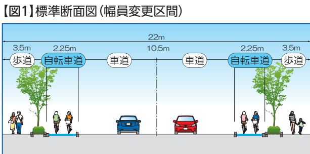
【図1】標準断面図(幅員変更区間) ※自転車道の整備形態については、今後、関係機関と調整し検討していきます。
