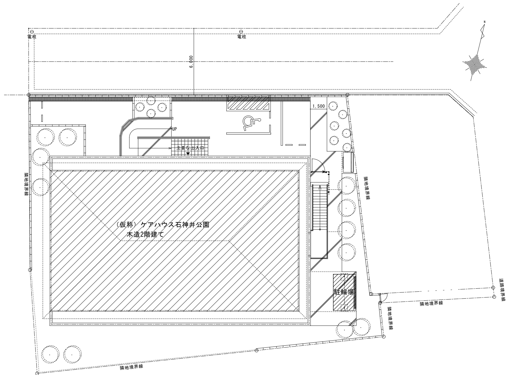
配置図（（仮称）ケアハウス石神井公園）
