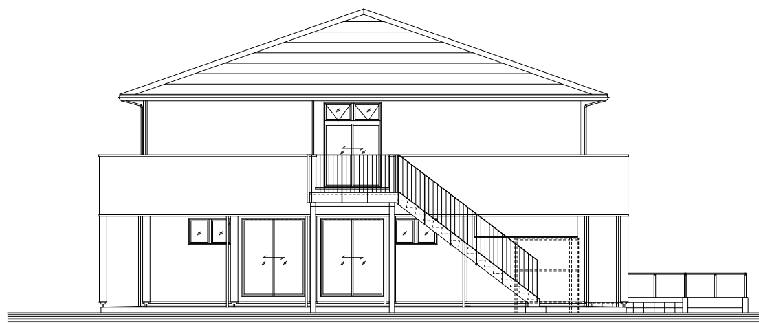
東側立面図
