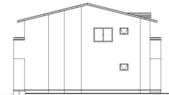
東側立面図
