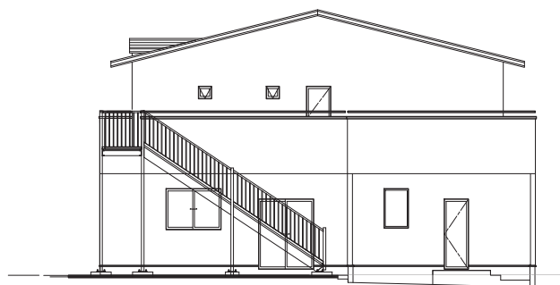
西側立面図
