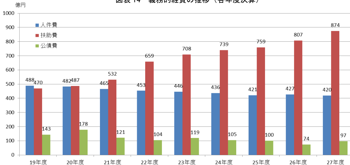
図表14 義務的経費の推移(各年度決算)
