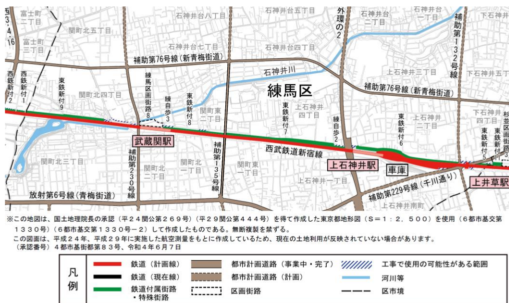
西武新宿線連続立体交差事業等の概略平面図
