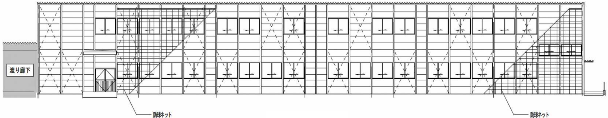
西側 立面図
