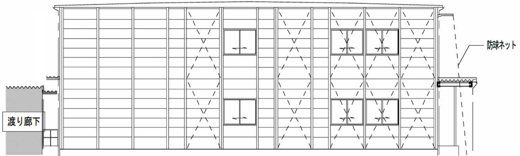
北側 立面図
