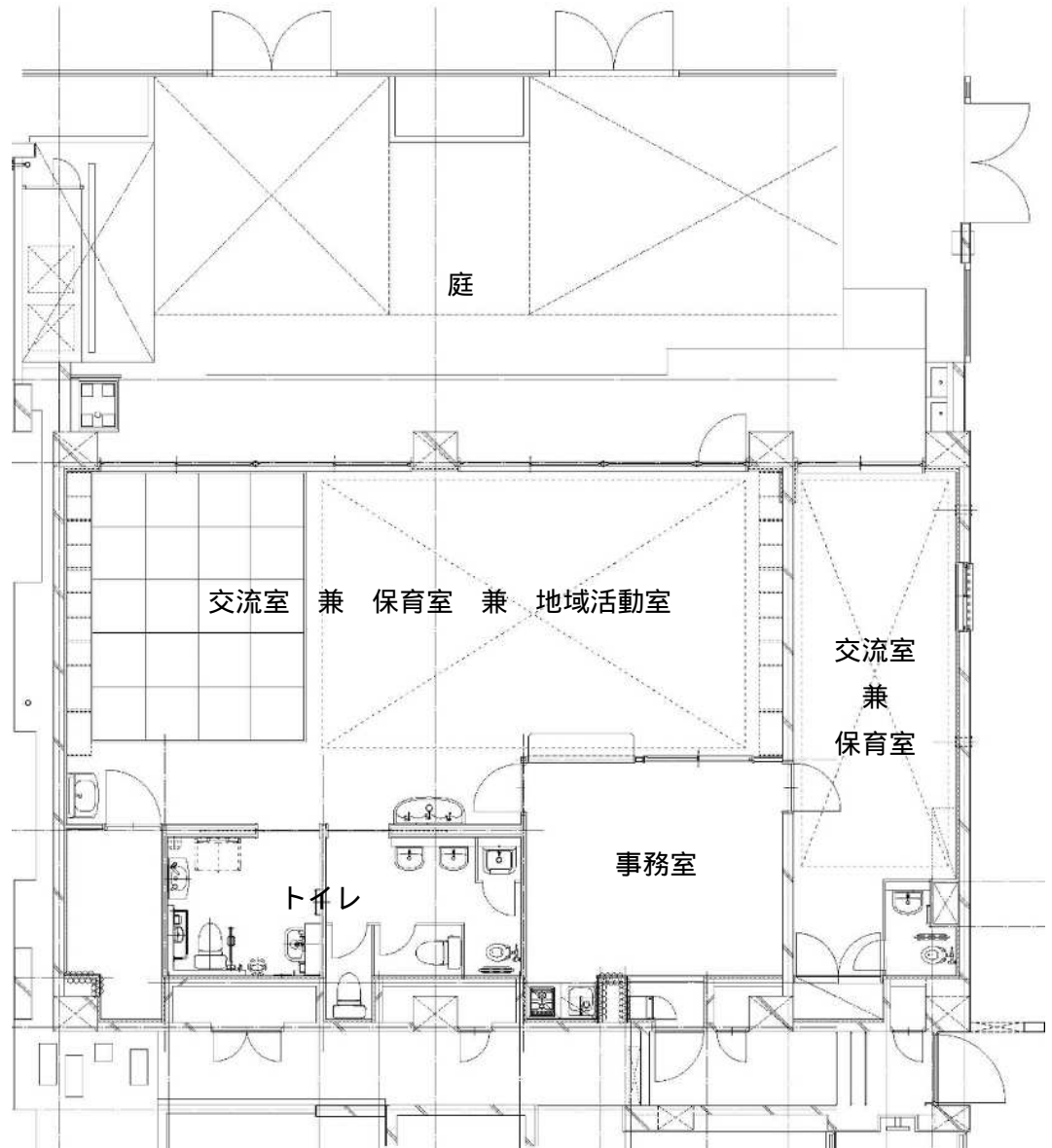
【平面図】
