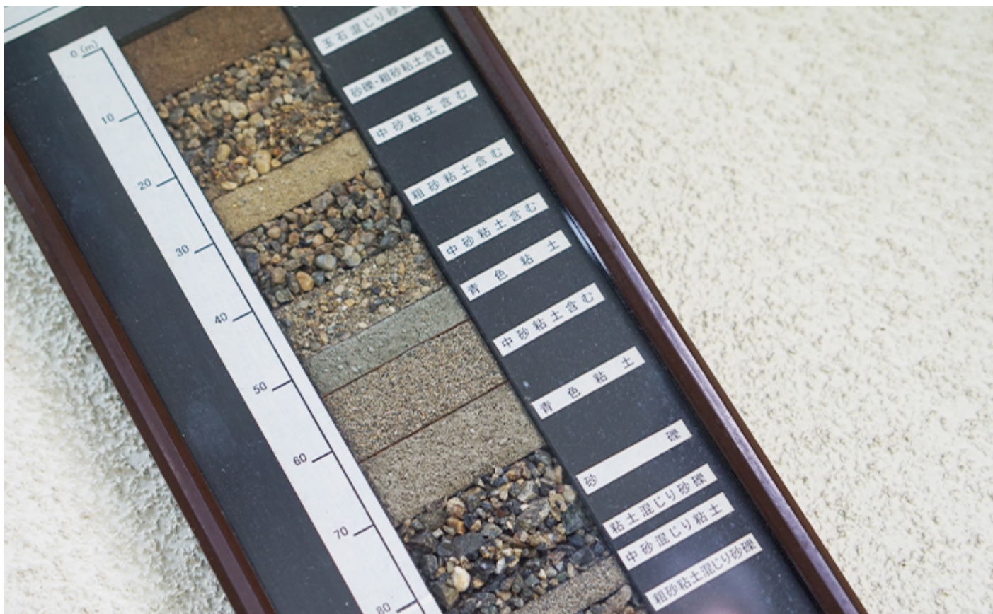
3号井戸が掘られた時の地層サンプル、一例ですが、何層もの地層で不純物がろ過され多くのミネラルを含む水になります
