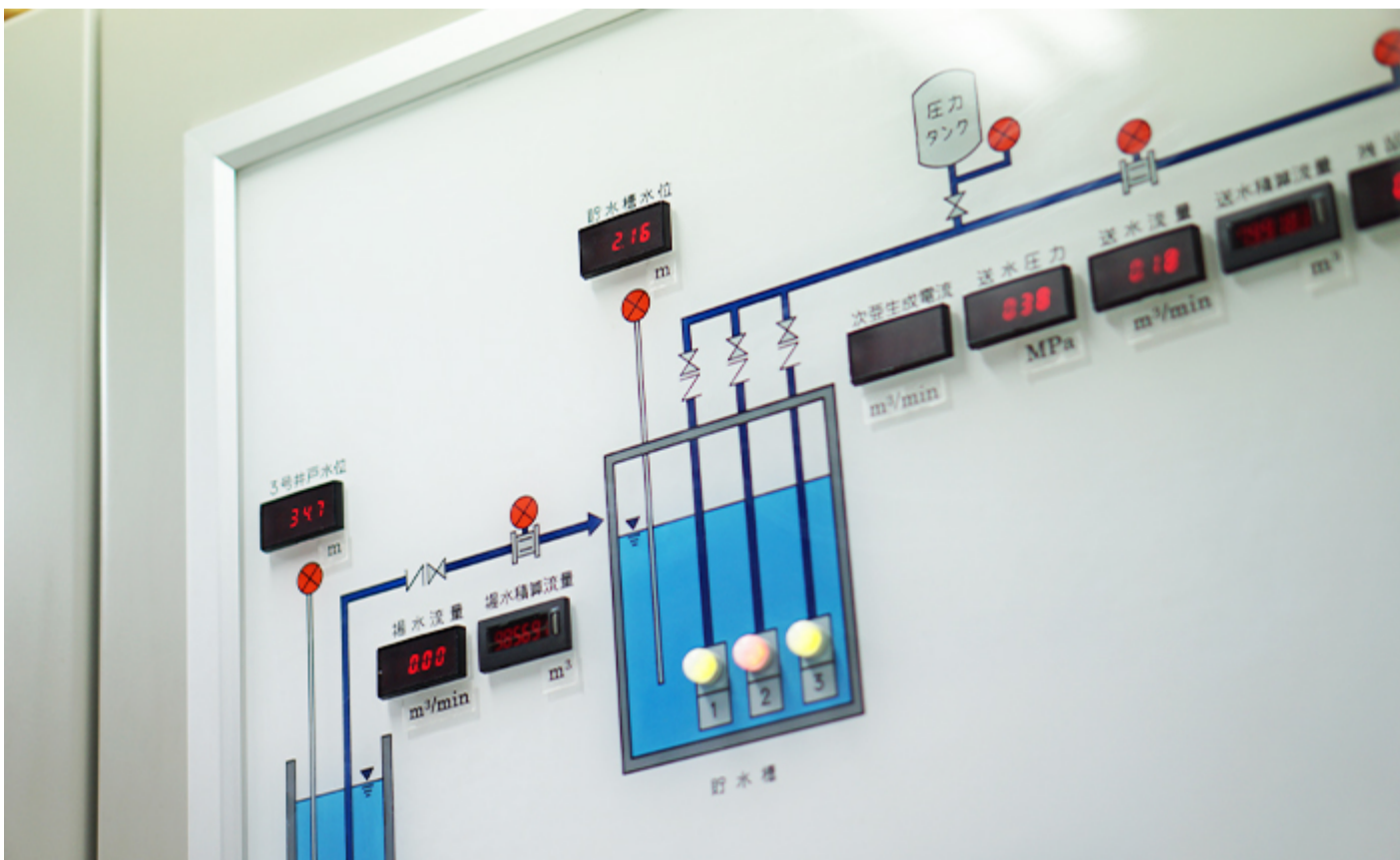
操作盤、赤いランプが稼働中の合図で 現在はNo2送水ポンプが稼働中
